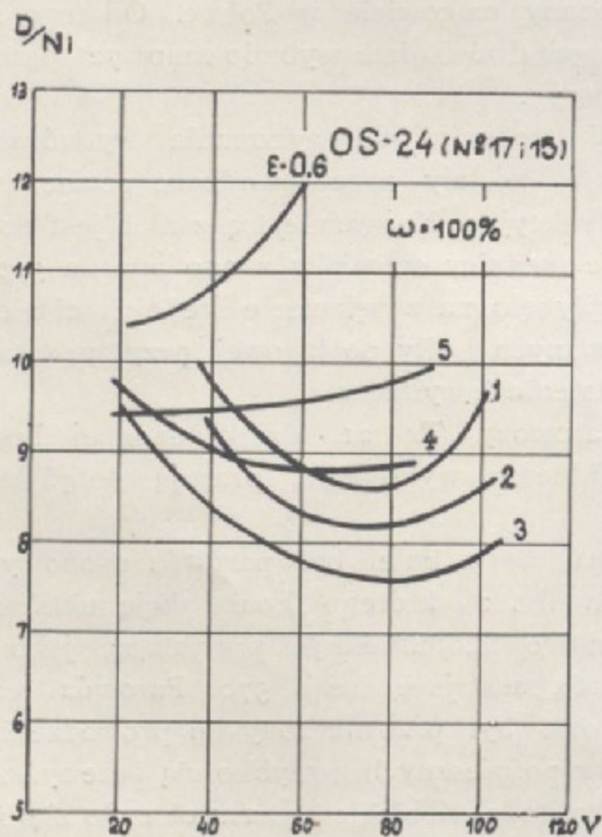
Fig. 3. Krzywe rozchodu pary na 1 KM i 1 godz. dla parowozu Os 24 ze stawidłem suwakowym.
