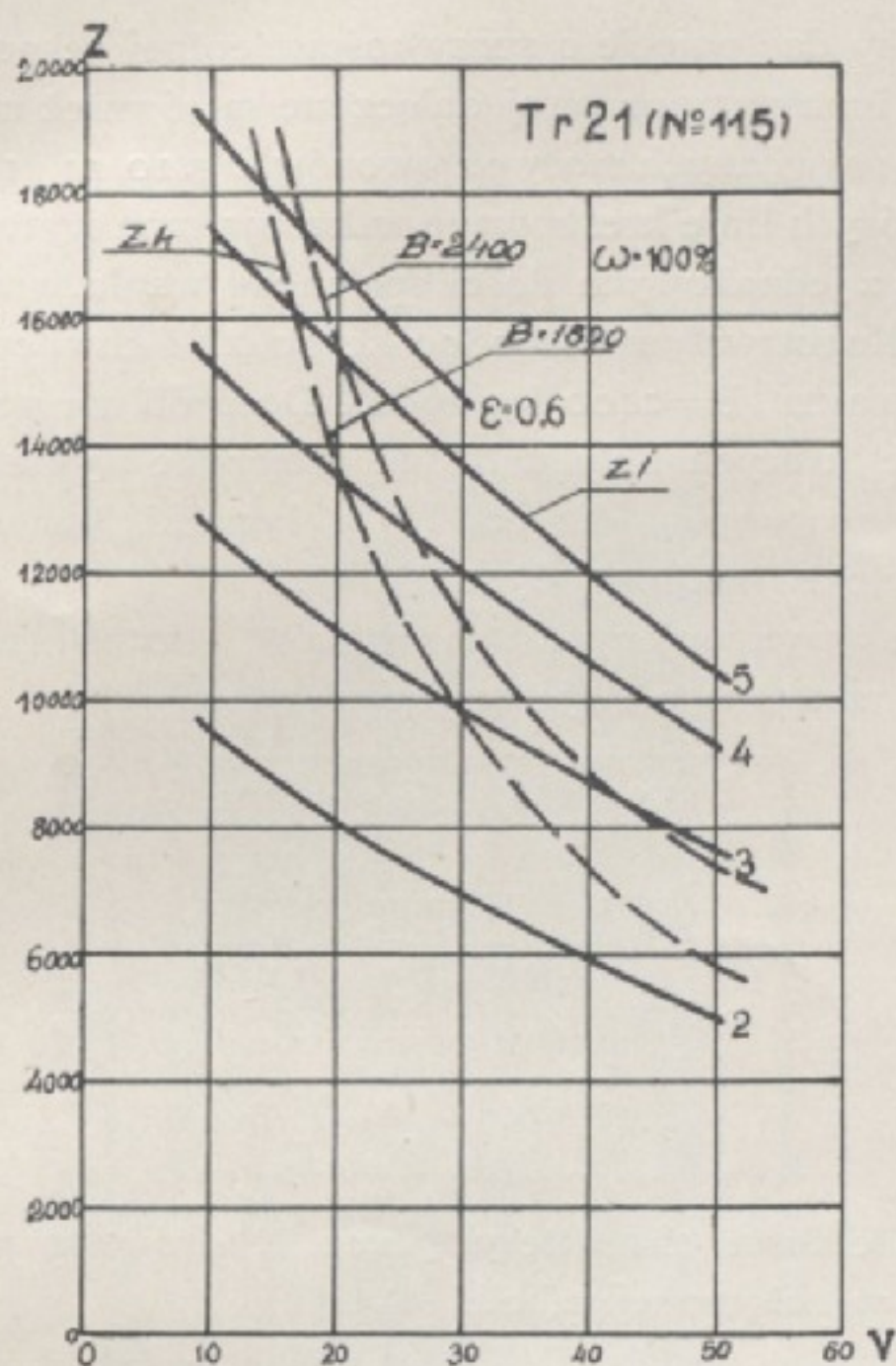
Fig. 7. Krzywe sił pociagowych cylindrowych i kotłowych dla parowozu Tr 21.
