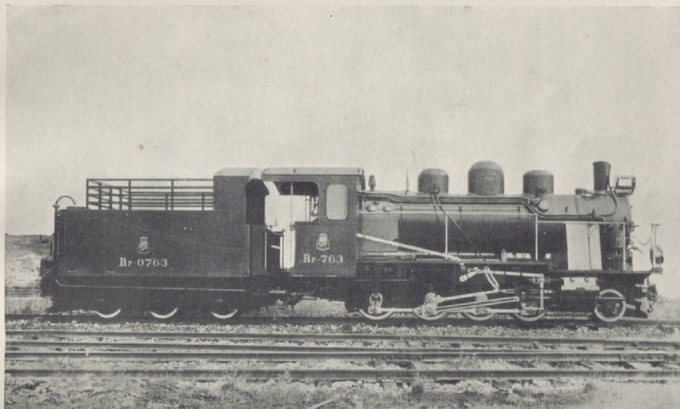
Parowóz na tor 750 mm dla Kolei Państwowych Łotewskich.
