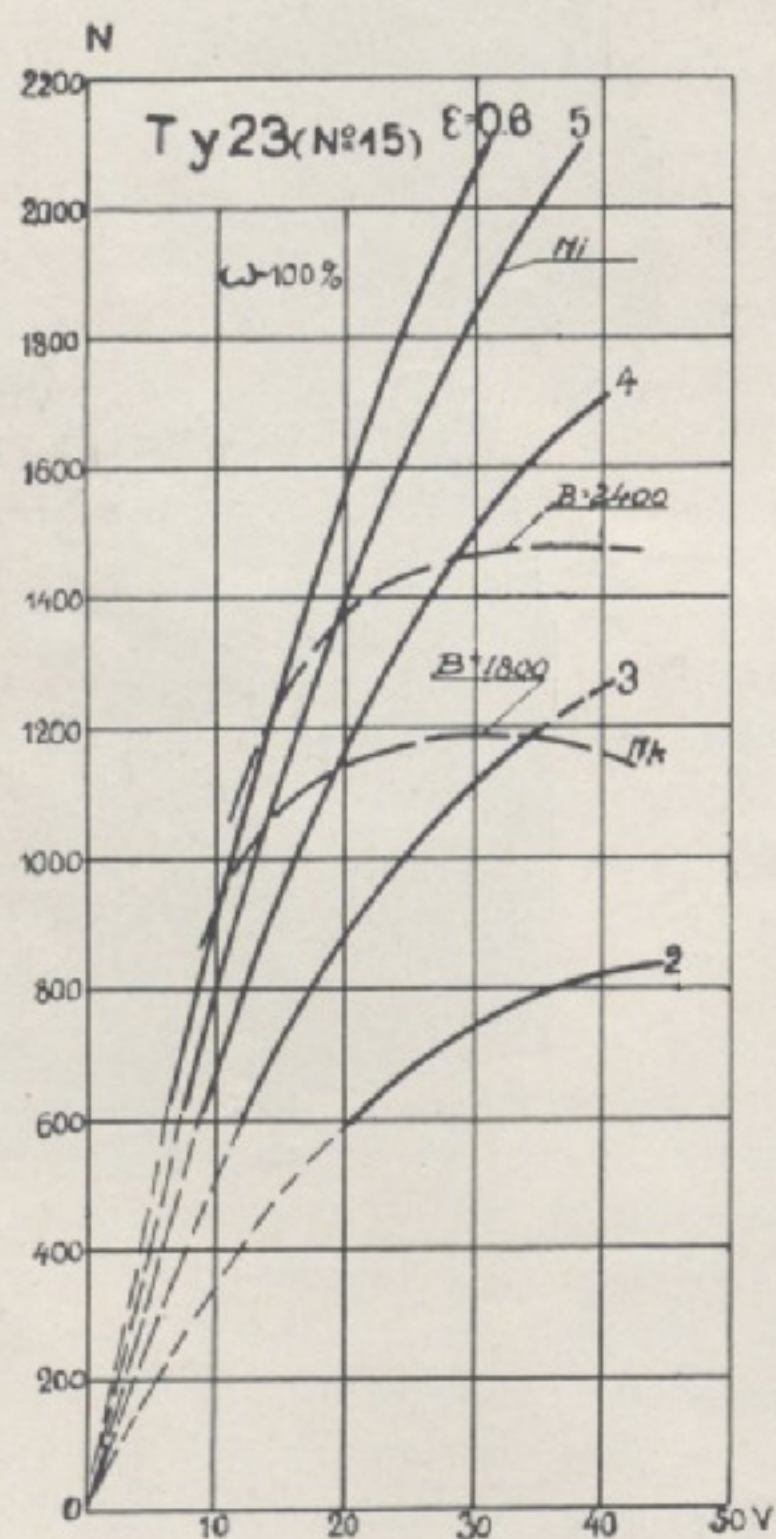
Fig. 12. Krzywe mocy parowozu Ty 23.
