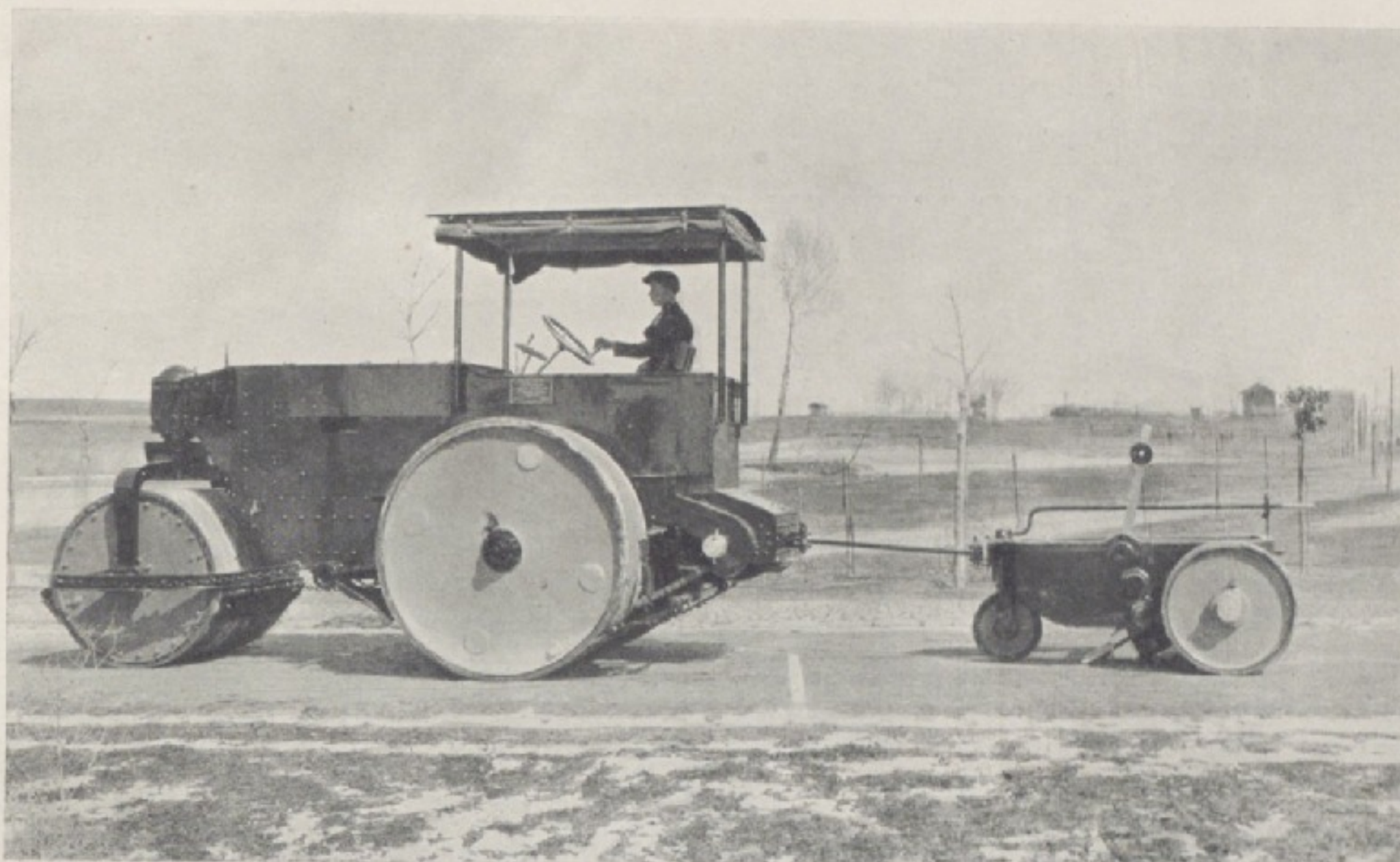
Fig. 17. Walec drogowy typu ciężki, o wadze 13.7/15.5 tonn, z rozrywaczem 3-oskardowym.
