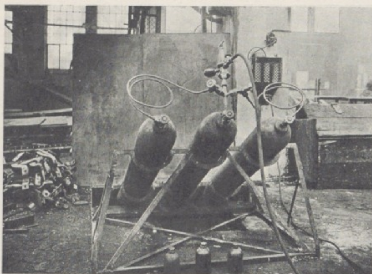
Fig. 4. Instalacja baterji butli tlenowych.
