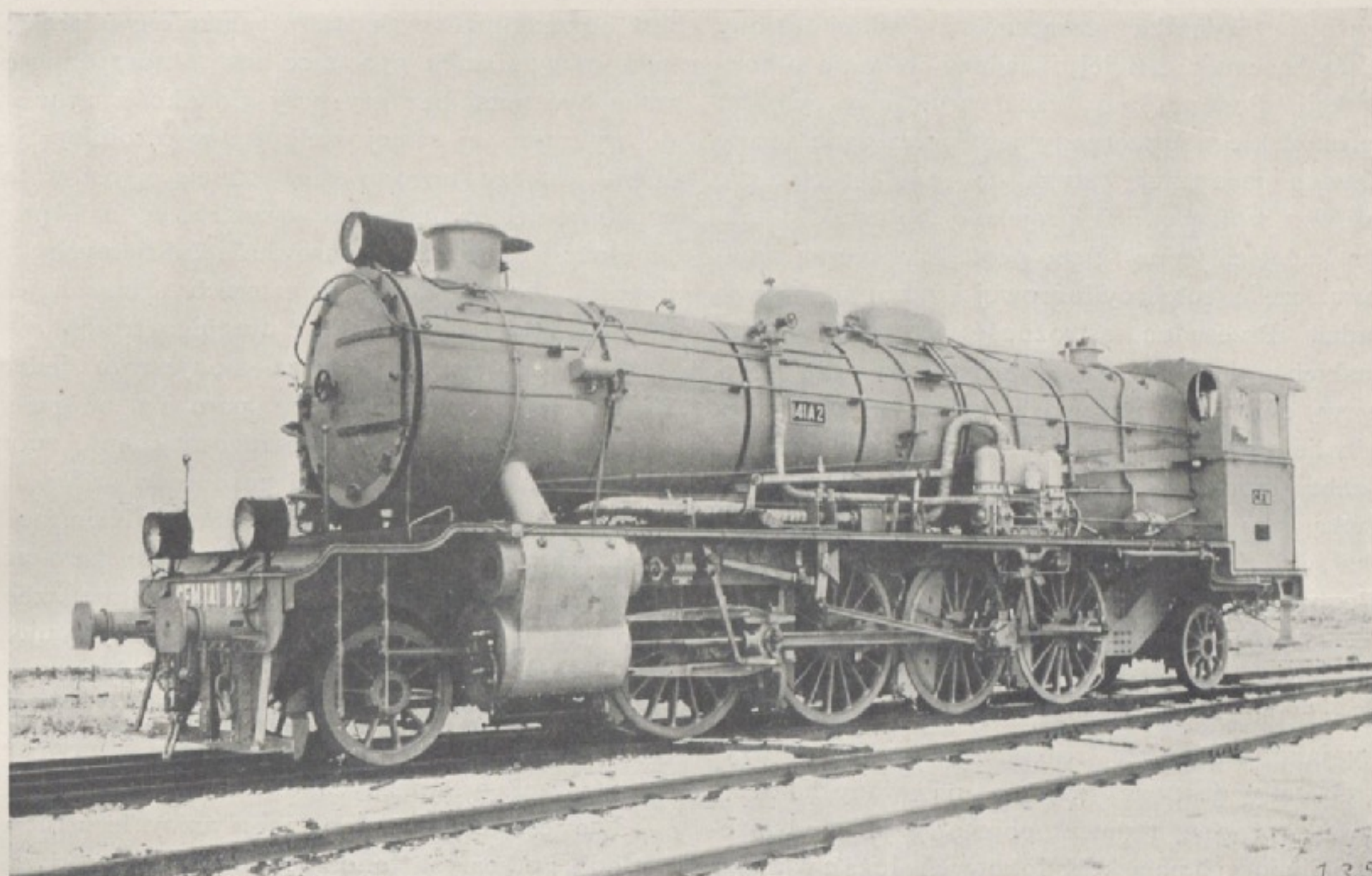
Parowóz osobowy 1—4—1 dla Towarzystwa Kolei Francuskich w Marokku.
