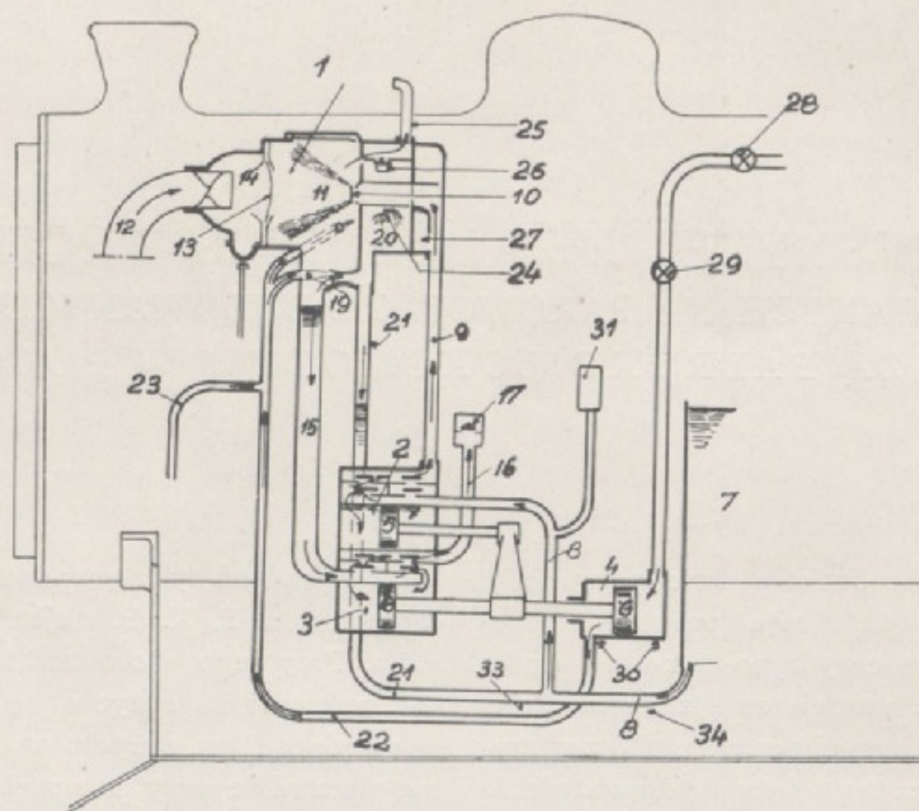
Fig. 1. Schemat pompy Worthingtona.
