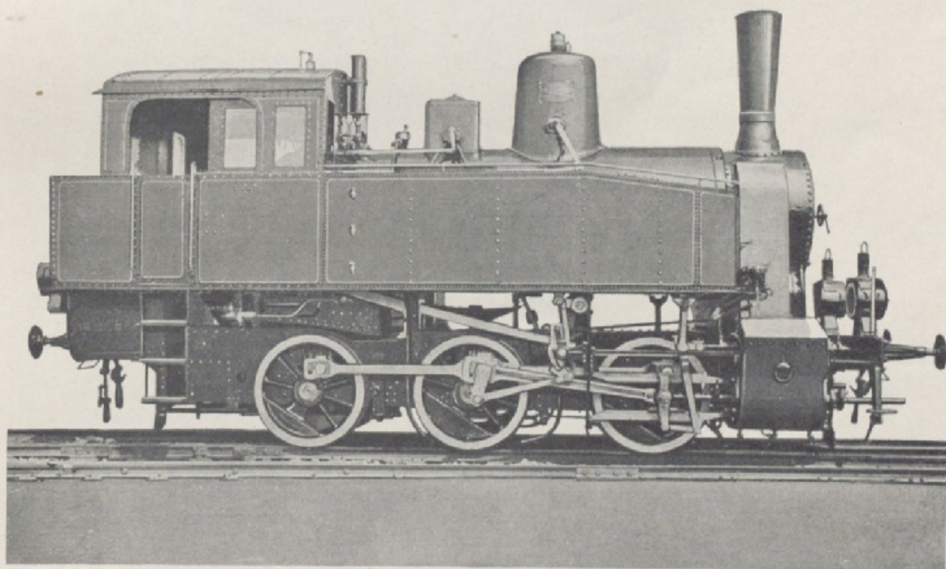
Fig. 14. Tenzrak 0-3-0 moc 450 KM normalnotor. na parę nasyc. lub przegrz.
