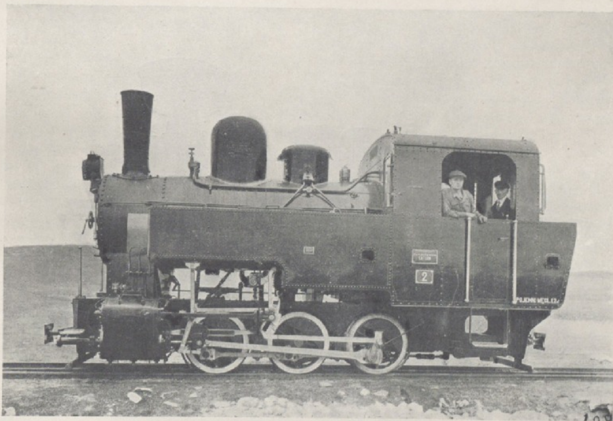
Fig. 10. Tendrzak 0—3—0 moc 225 KM szer. toru 1000 m/m.
