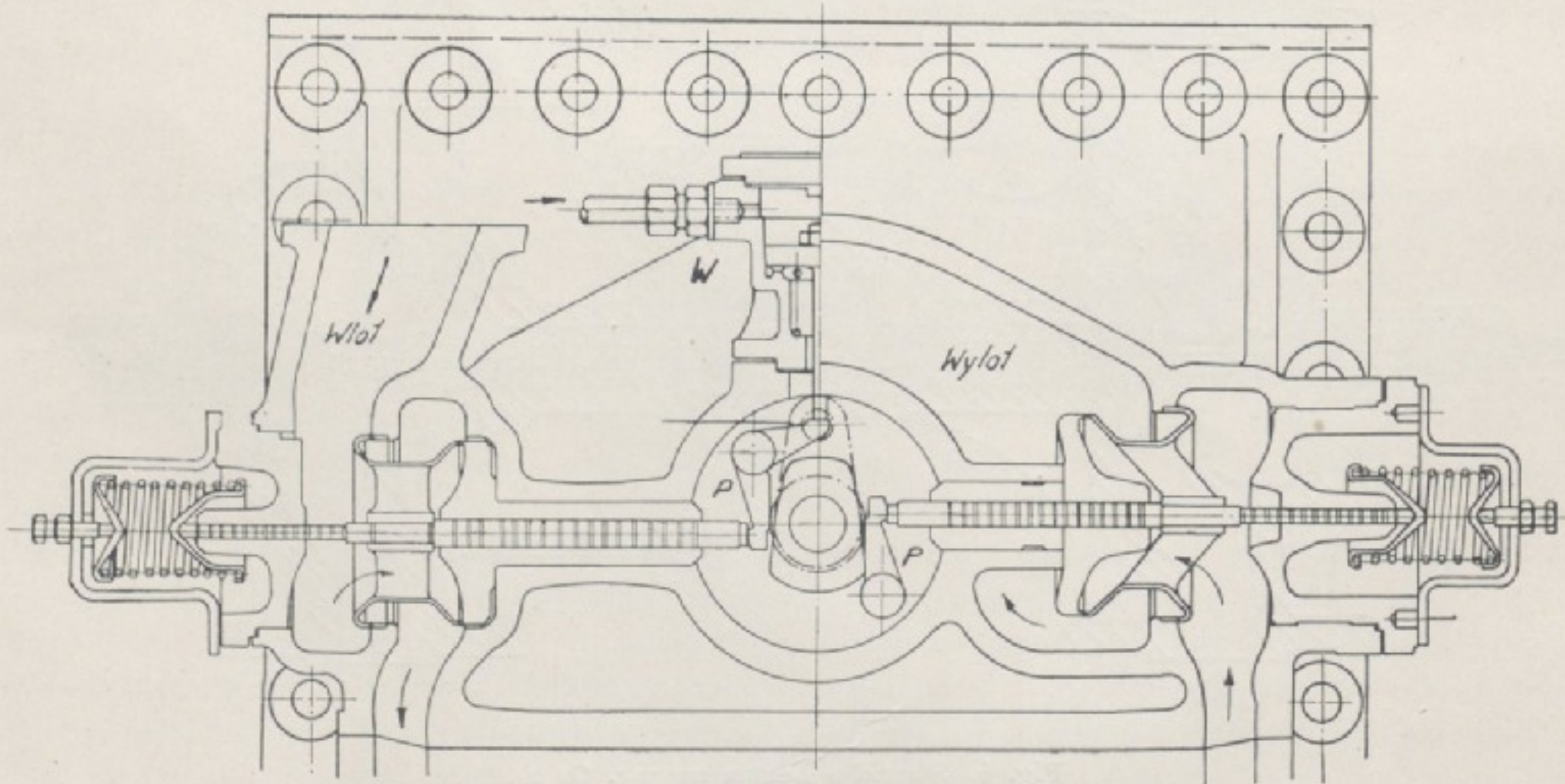
Fig. 8. Zaworowe stawidło Lentza na par. Ok22.
