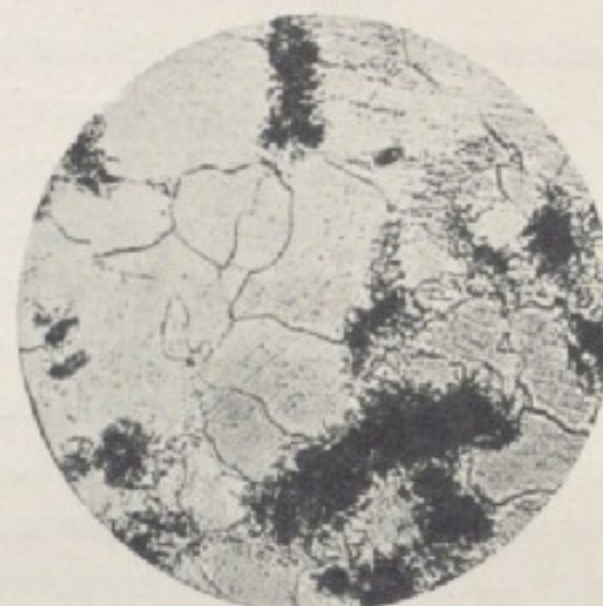
Mikrofotogr. 4. \times 250 .
