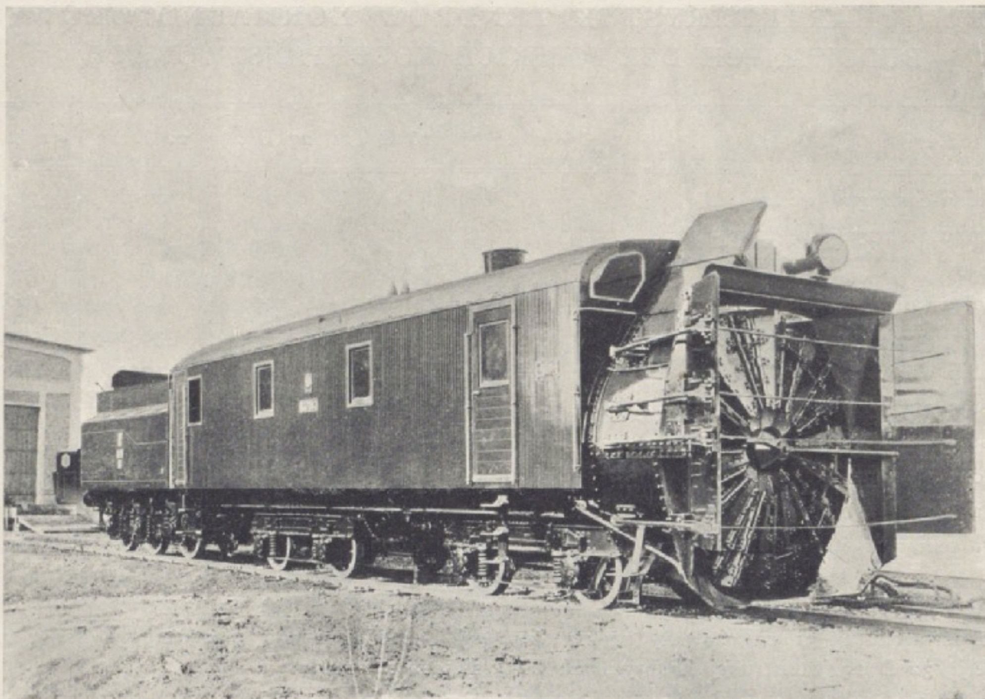
Fig. 14. Wirowy pług odśnieżny systemu «Nydquist i Holm».
