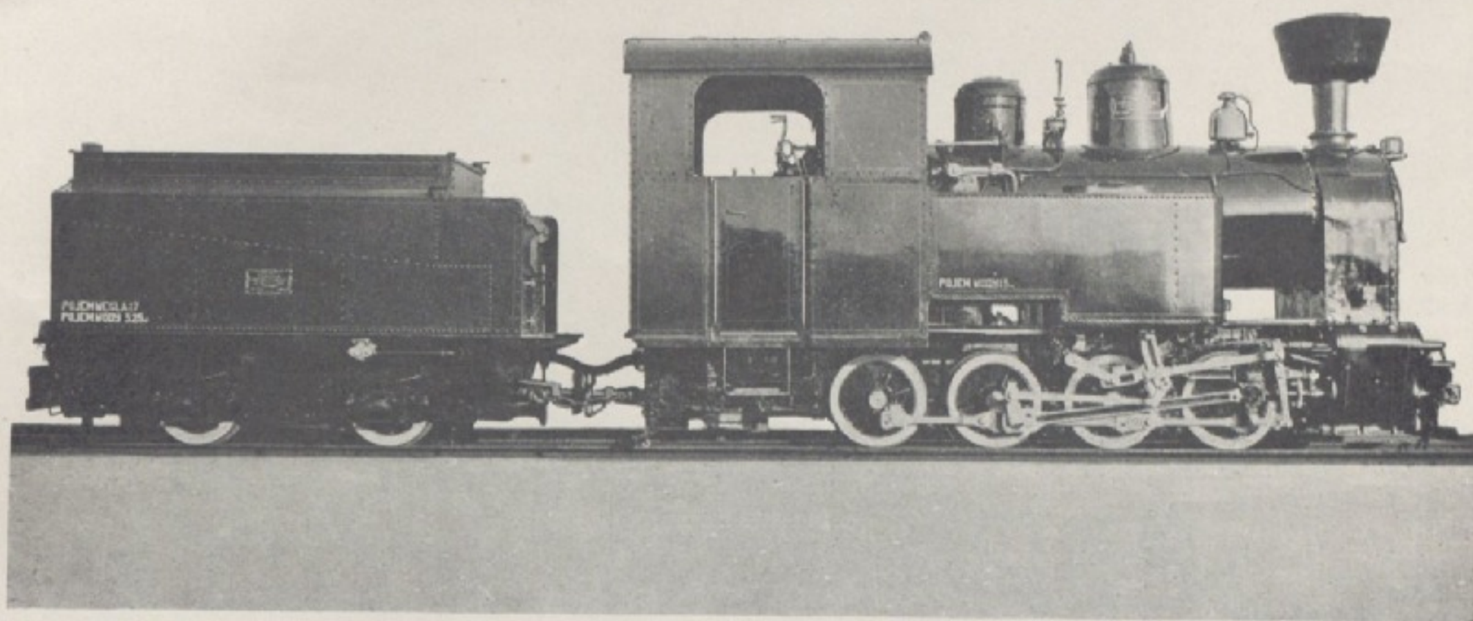
Fig. 9. Parowóz 0—4—0 moc 110 KM szer. toru 600 m/m z tendrem 2-osiowym.
