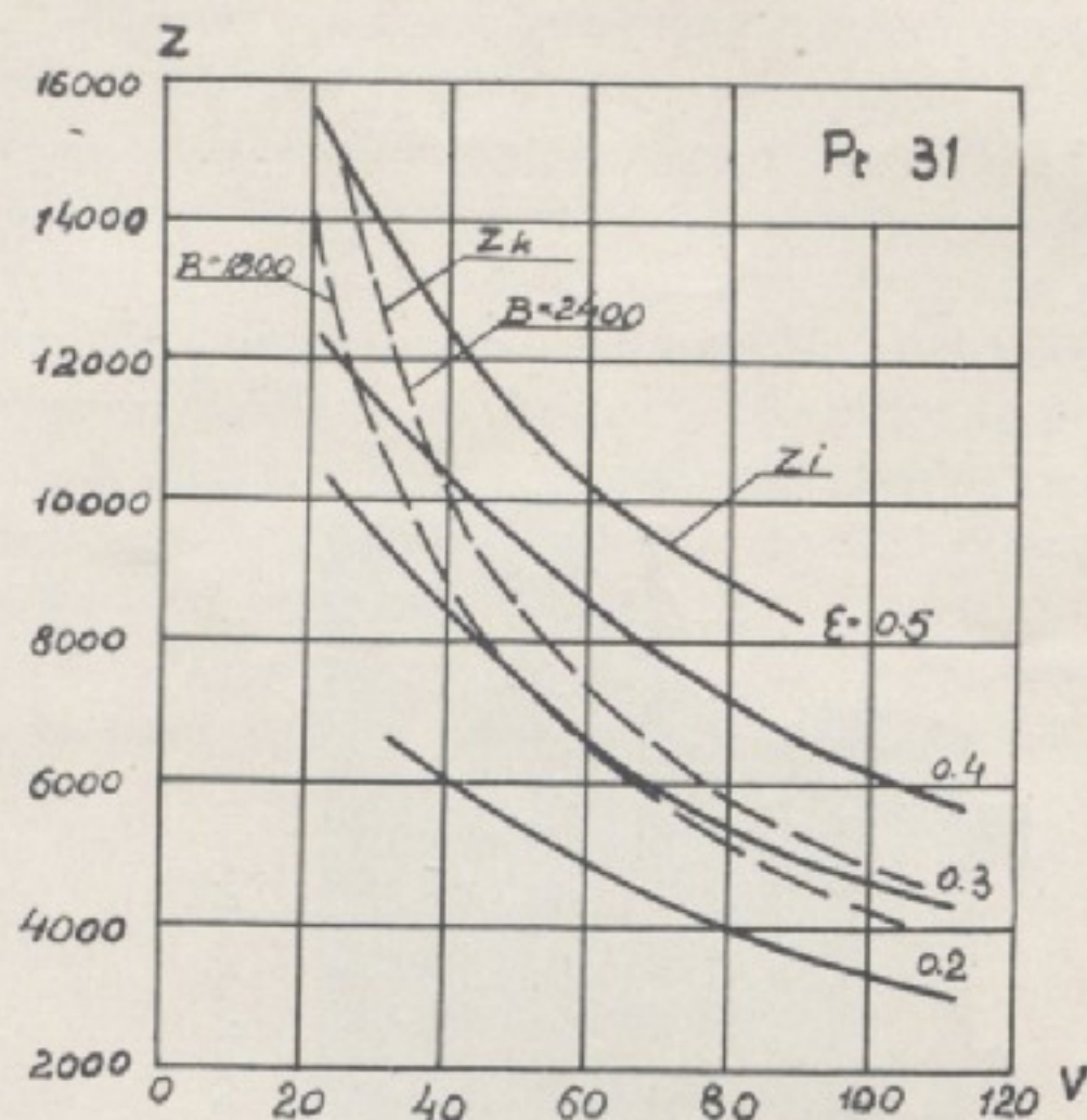
Fig. 13. Przypuszczalne krzywe sił pociagowych cylindrowych i kotłowych dla parowozu Pt 31.
