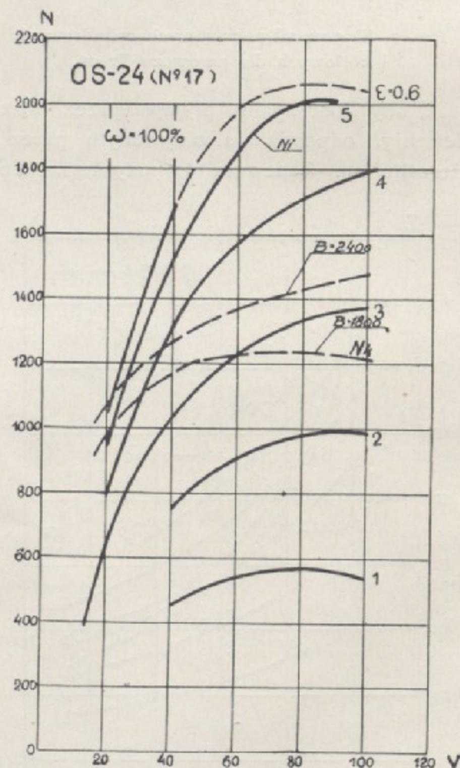
Fig. 11. Krzywe mocy parowozu Os 24 ze stawidłem suwakowym.
