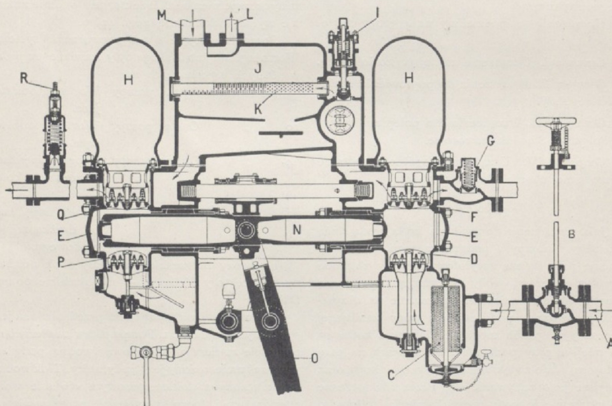
Fig. 2. Pompa zasilająca «Dabeg».
