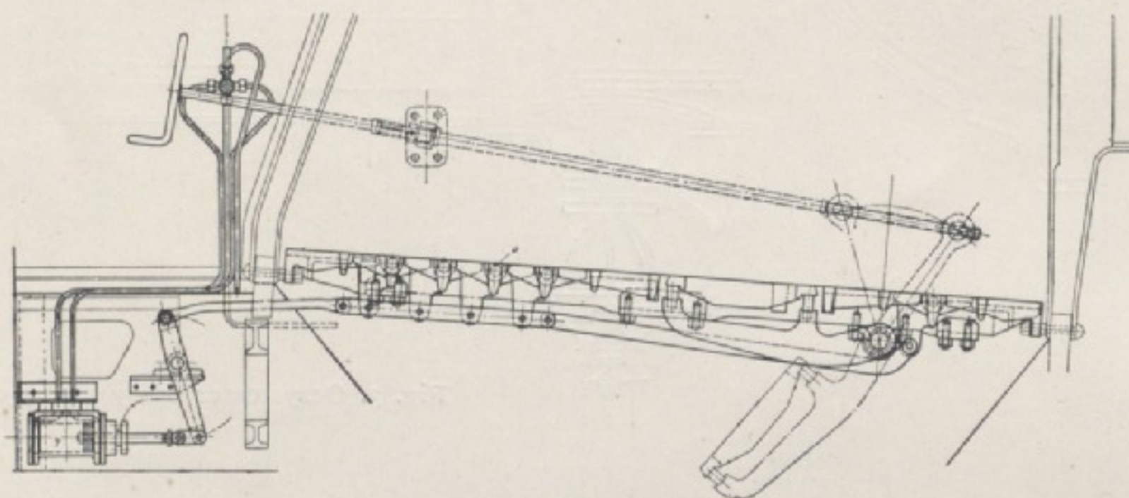
Fig. 4. Ruszt wstrząsany.
