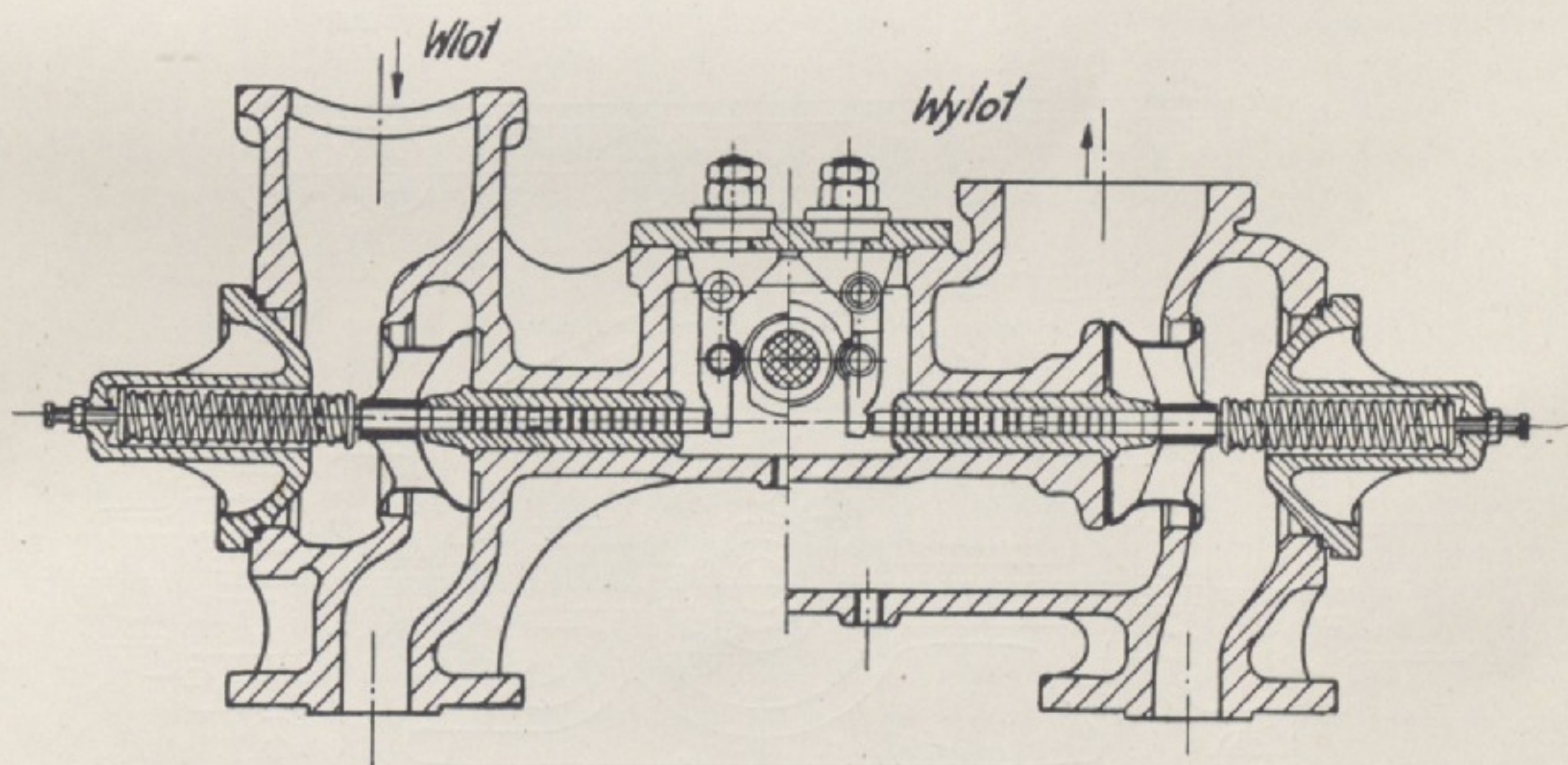
Fig. 6. Stawidło Lentza na par. Os 24.
