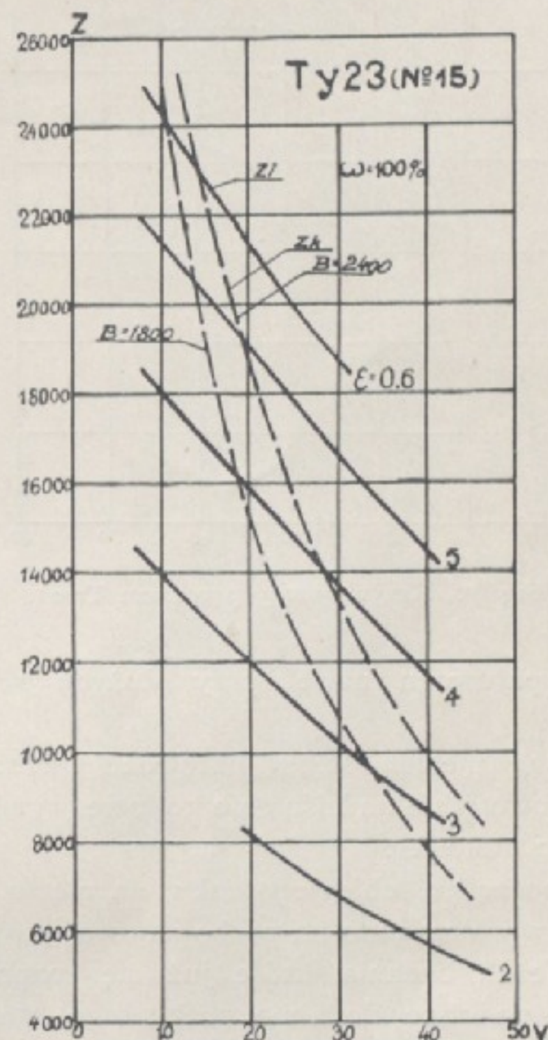
Fig. 9. Krzywe sił pociagowych cylindrowych i kotłowych dla parowozu Ty 23.
