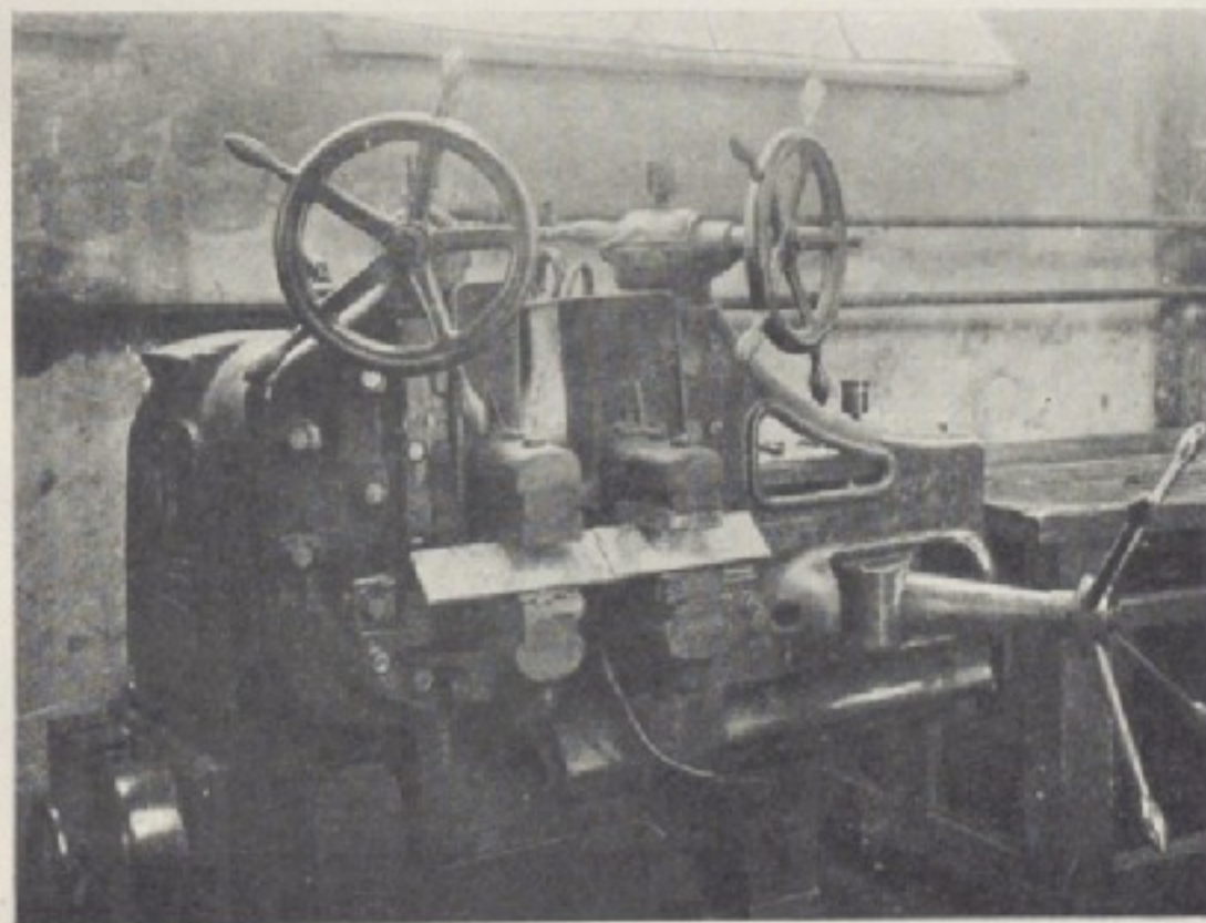
Fig. 5. Maszyna do spawania stykowego.
