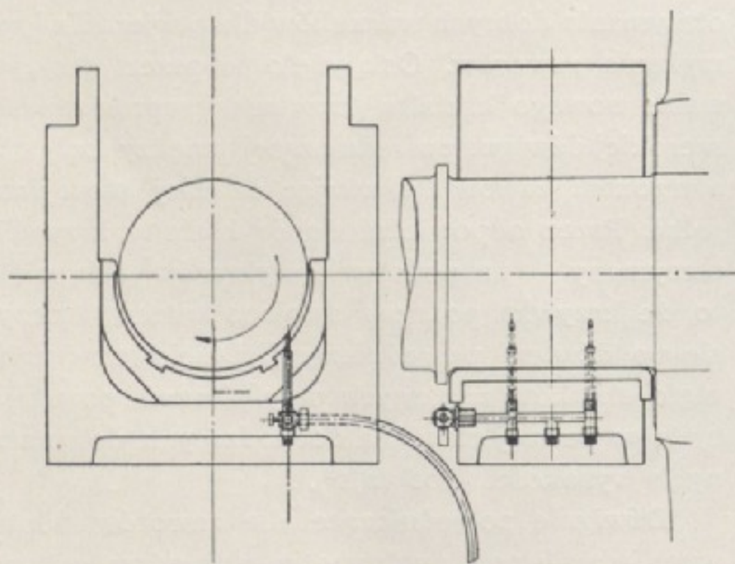
Fig. 11. Doprowadzenie smaru do maźnicy.
