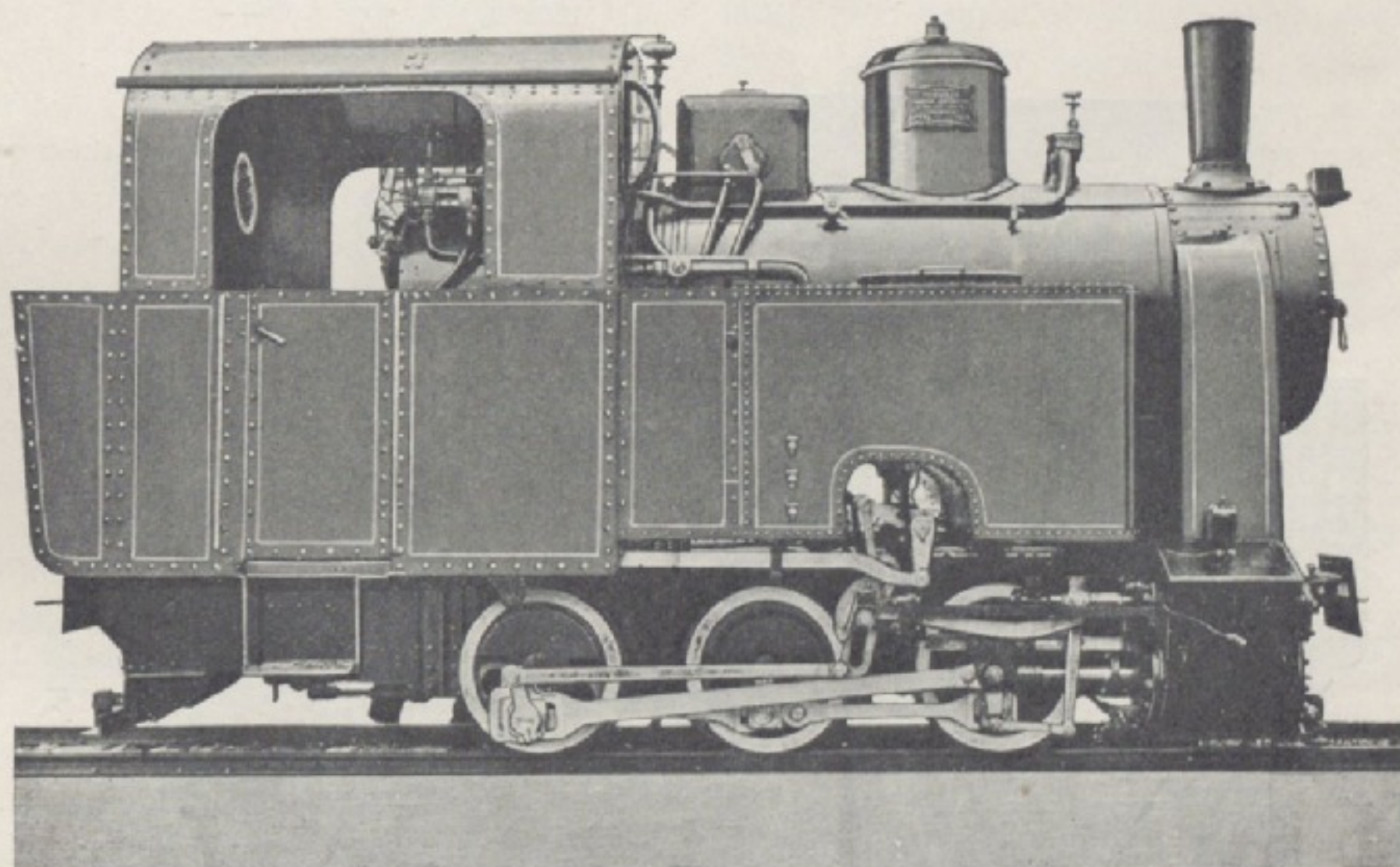
Fig. 2. Tendrzak 0—3—0 moc 90 KM szer. toru 750 i 800 m/m.
