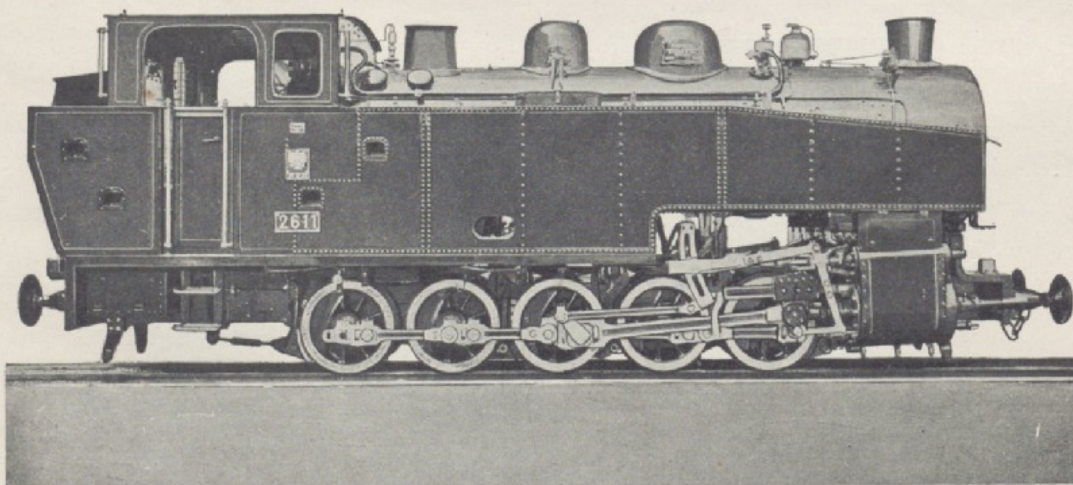
Fig. 8. Tenzak 0—5—0 moc 400 KM szer. toru 785 m/m na parę przegrzaną (Typ «Górnośląski»).
