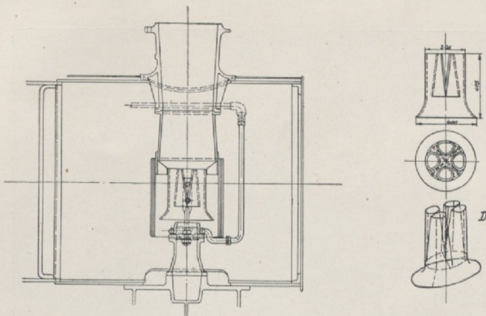
Fig. 5. Urządzenie cięgowe «Kylchap».
