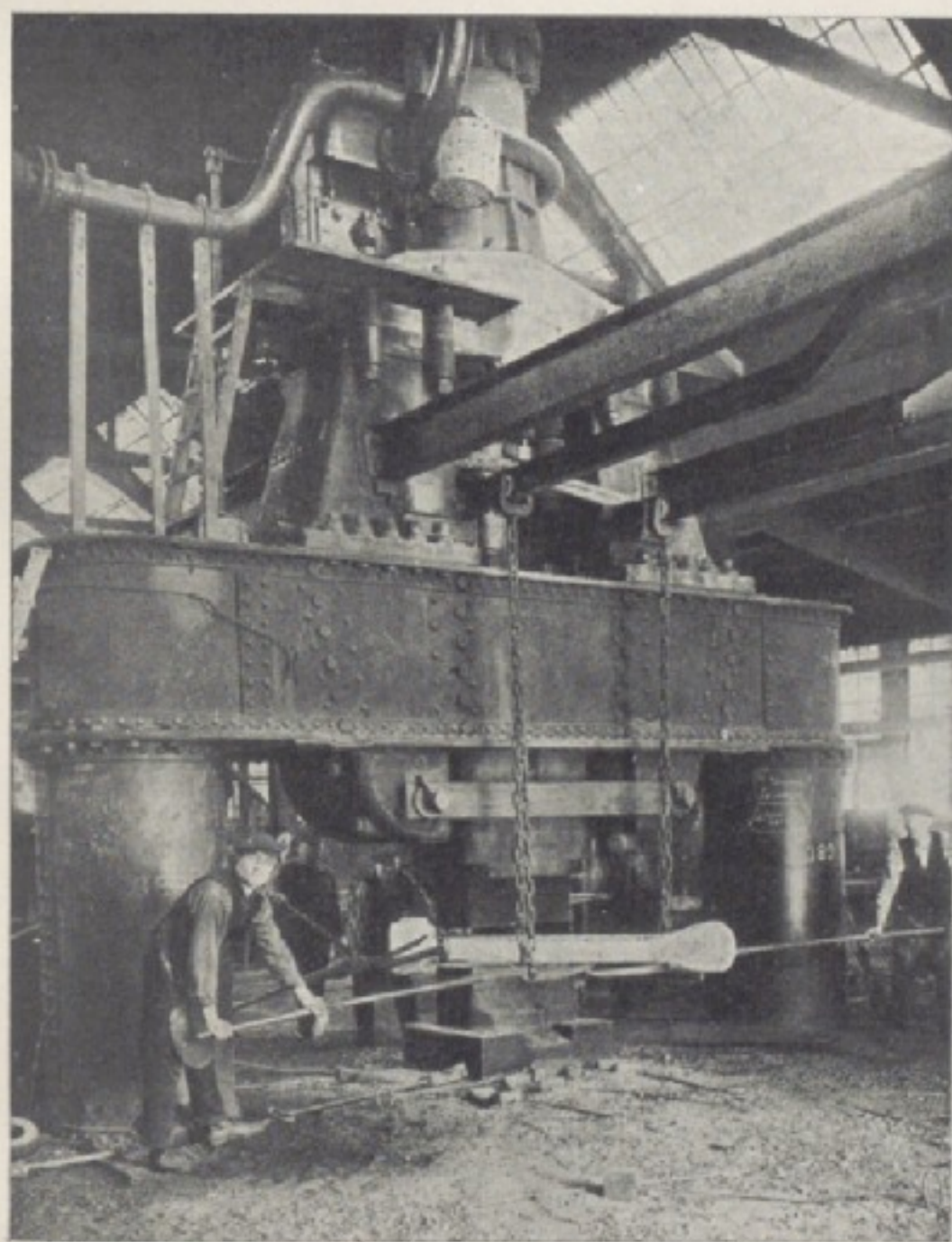
Fig. 3. Kucie korbowodu pod powietrznym młotem 5000 kg.
