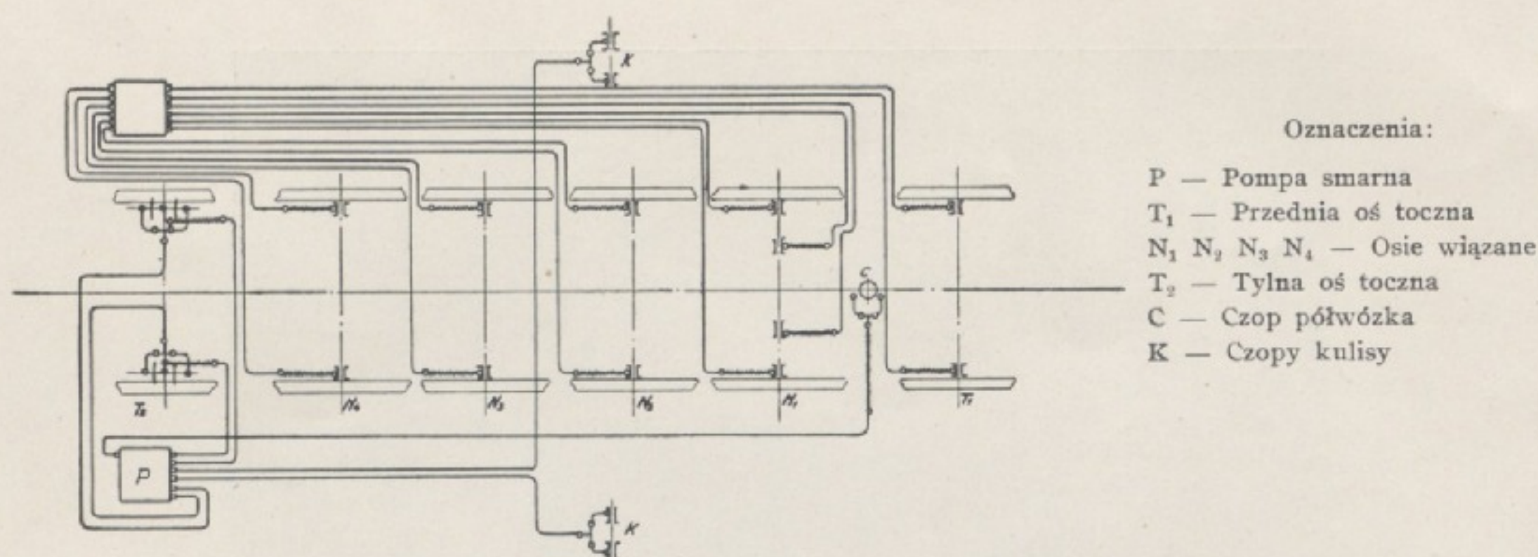
Fig. 10. Układ rurociągów dla centralnego smarowania maźnic.
