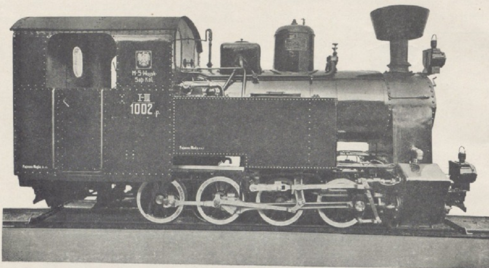
Fig 3. Tenzrak 0-4-0 moc 100 KM szer. toru 600/750 m/m.
