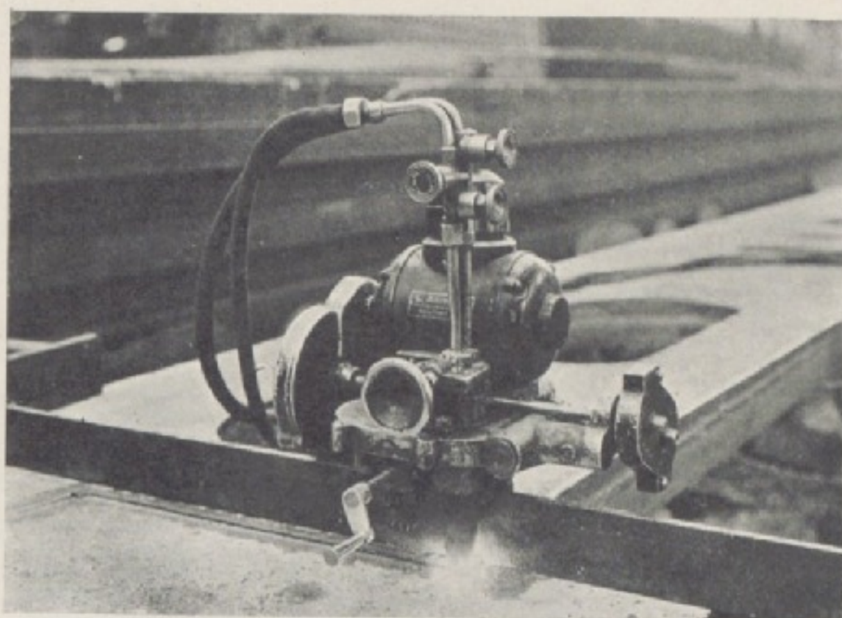
Fig. 2. Maszyna do cięcia grubych blach.
