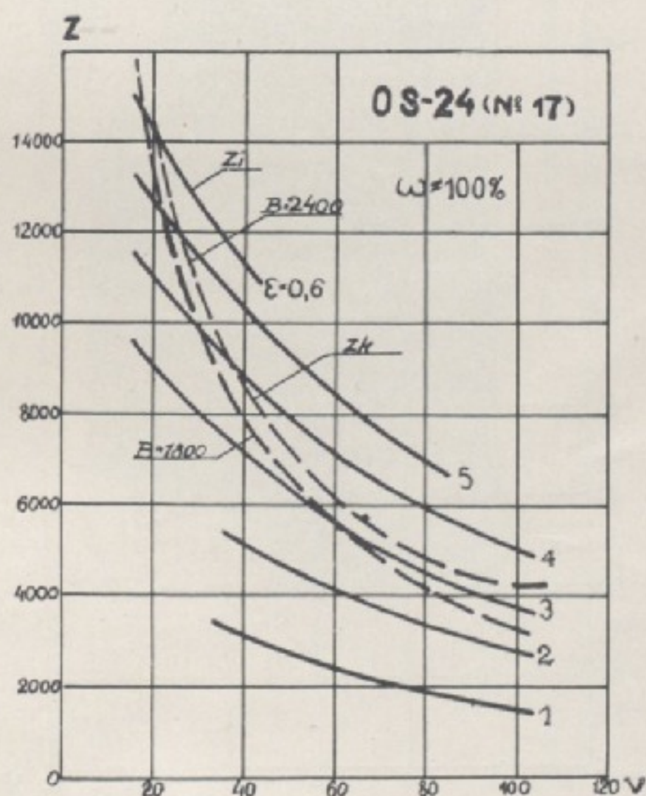
Fig. 8. Krzywe sił pociagowych cylindrowych i kotłowych dla parowozu Os 24.
