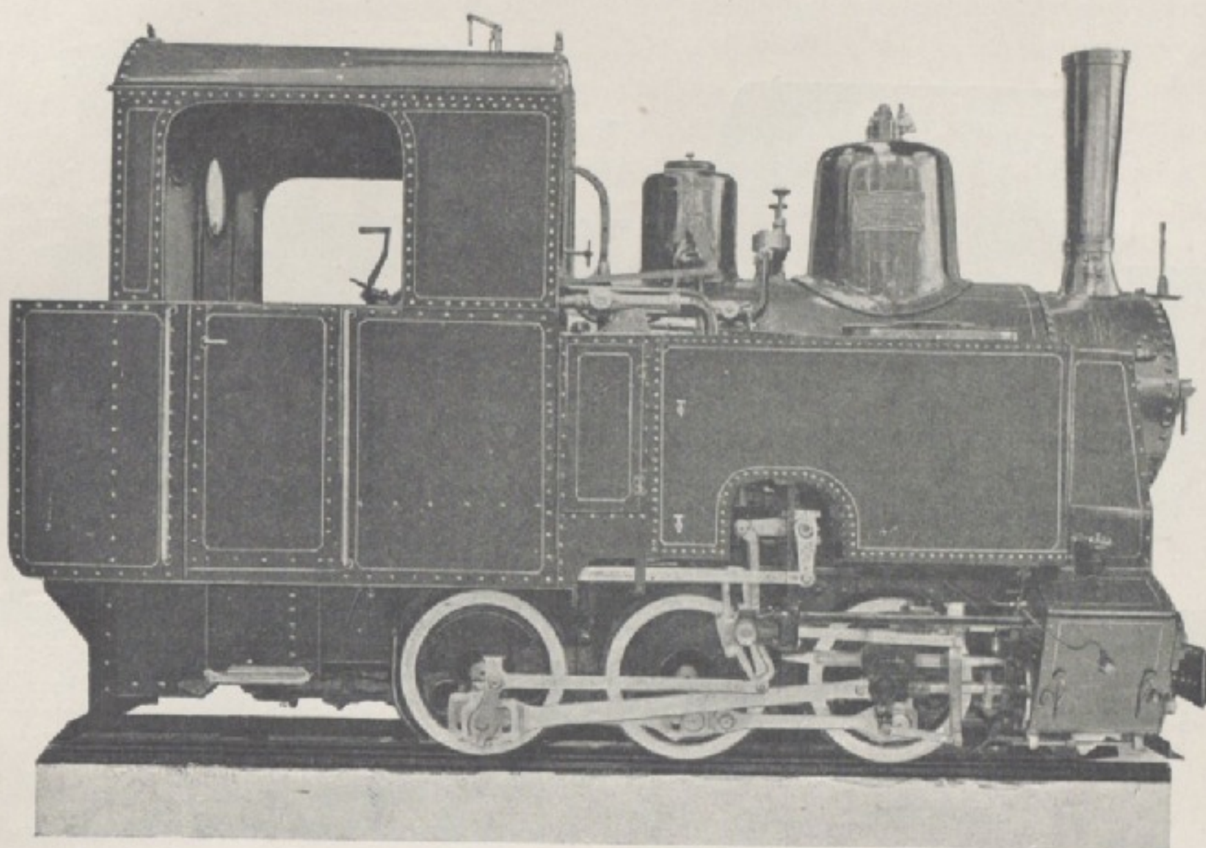
Fig. 5. Tendrzak 0—3—0 moc 60 KM szer. toru 600 i 750 m/m.
