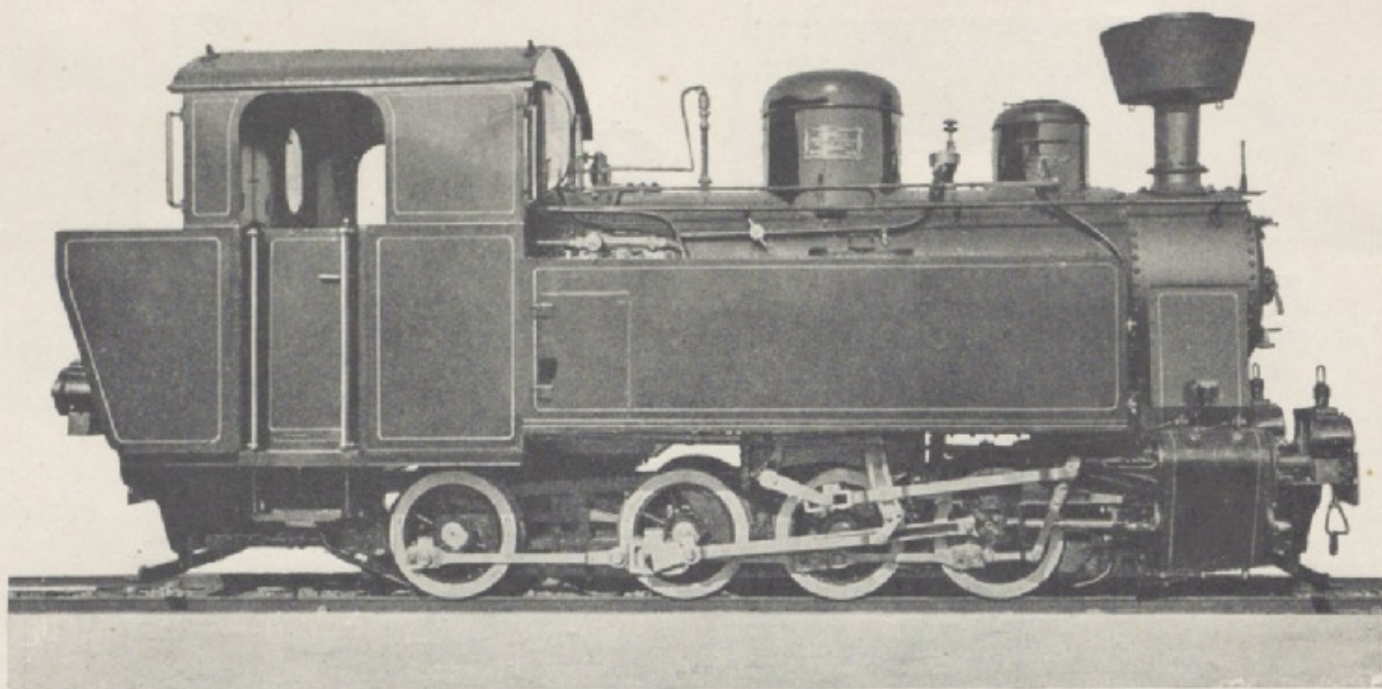
Fig. 7. Tenzak 0—4—0 moc 110 KM. szer. toru 750 m/m (Typ «Wisła»).
