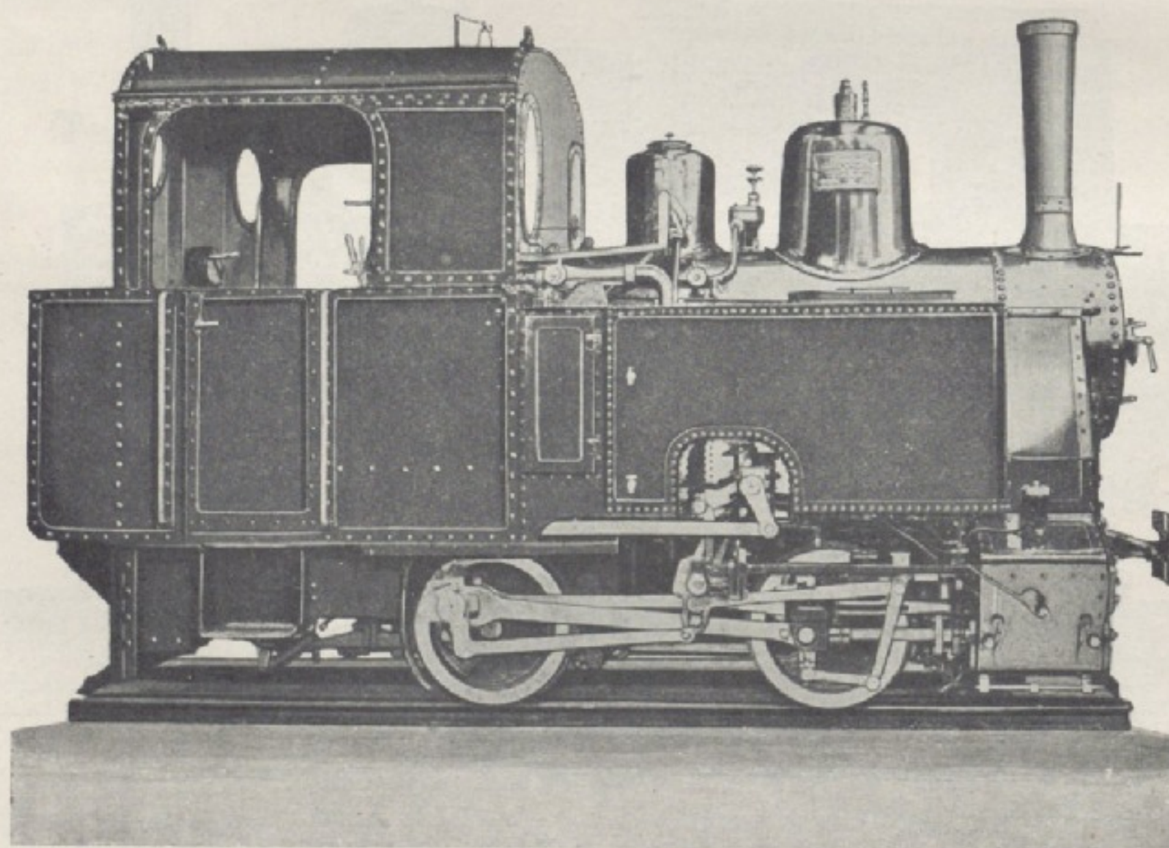
Fig. 4. Tenzrak 0-2-0 moc 60 KM szer. toru 800 m/m.
