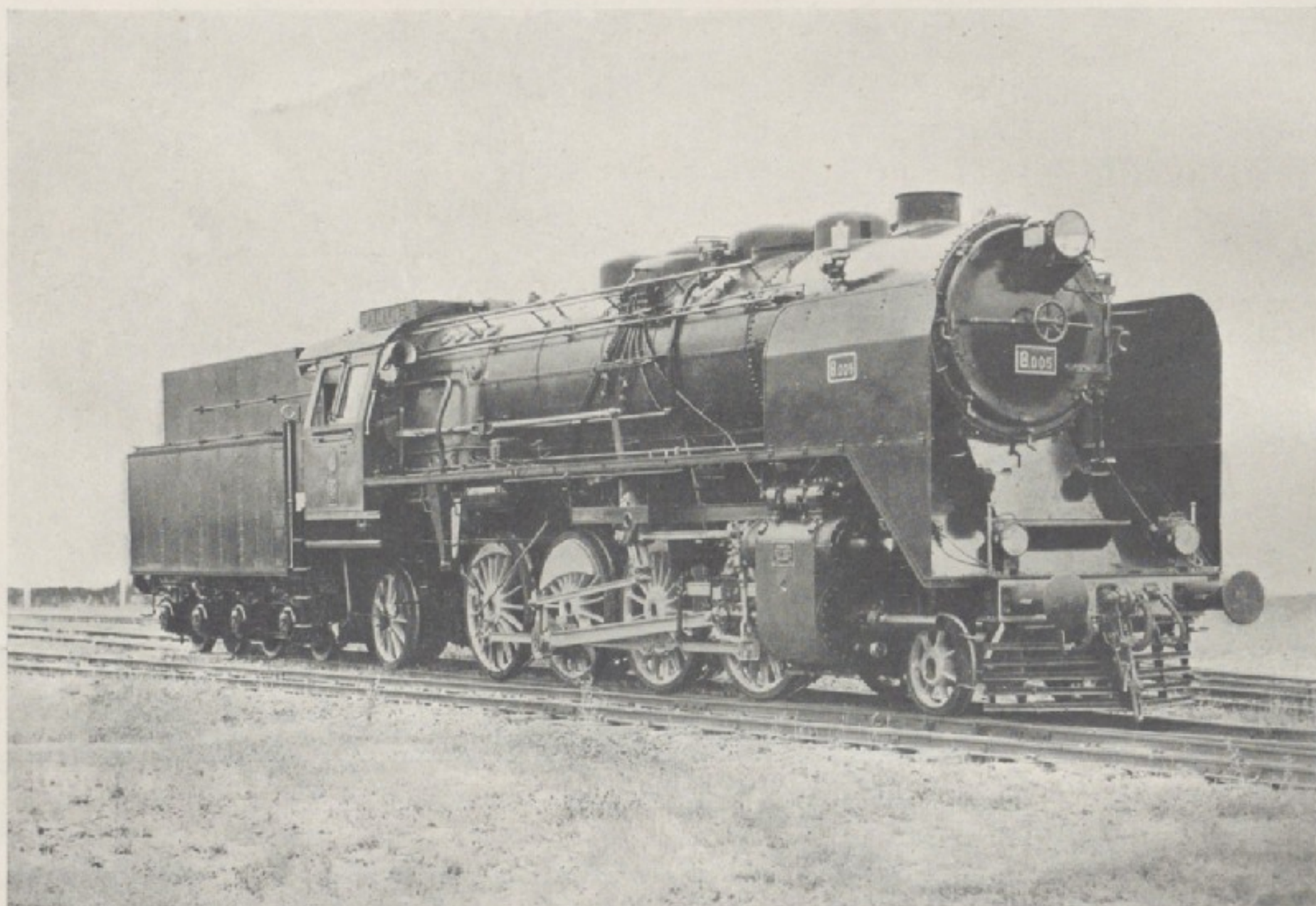
Parowóz pospieszny 1-4-1 dla Bułgarskich Kolei Państwowych.
