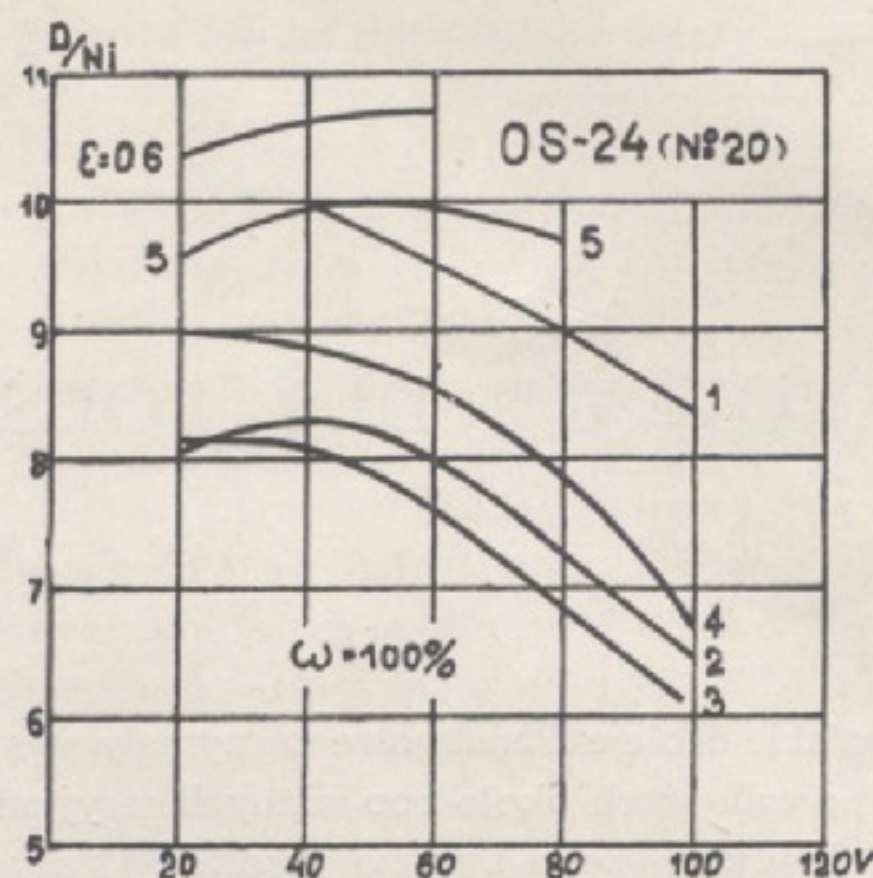
Fig. 4. Krzywe rozchodu pary na 1 KM i godz. dla parowozu Os 24 ze stawidłem zaworowym.
