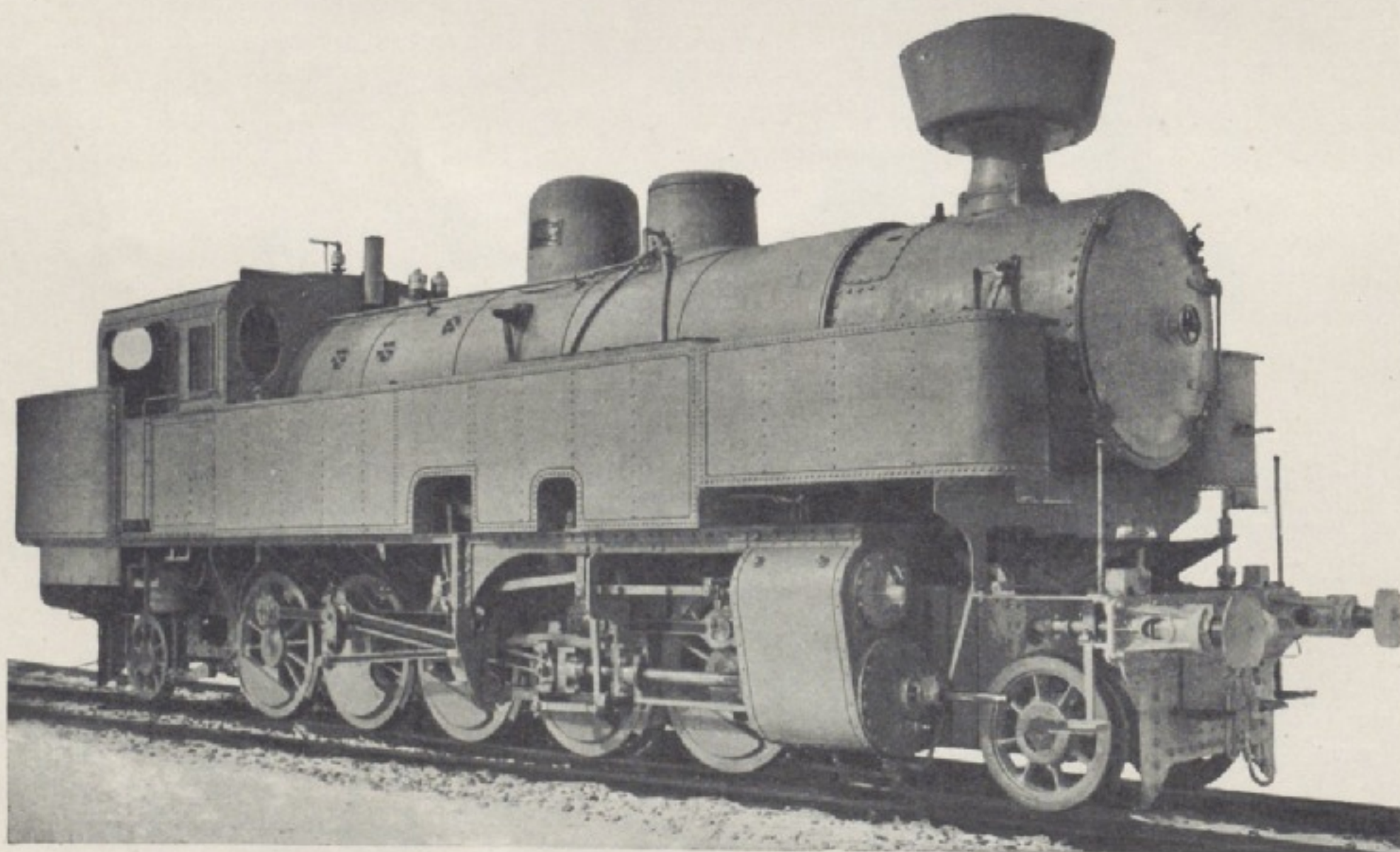
Fig. 12. Tendrzak 1—5—1 moc 950 KM normalnotor. na parę przegrzaną.
