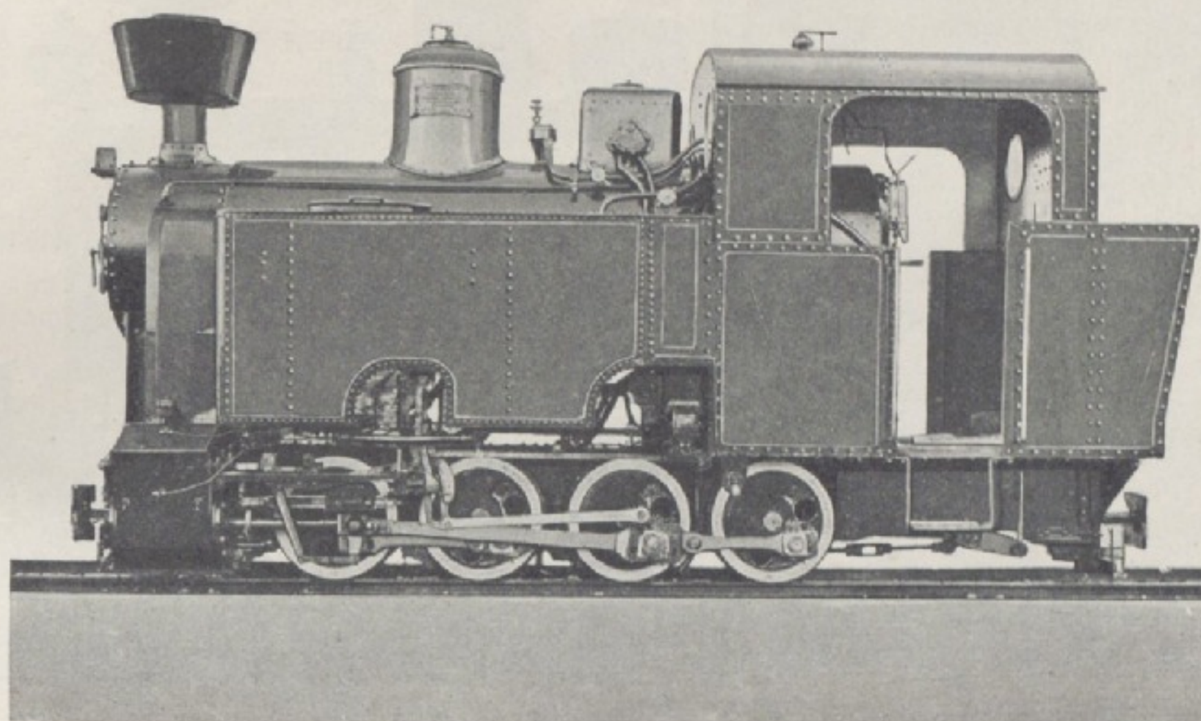
Fig. 1. Tendrzak 0—4—0 moc 120 KM szer. toru 600 i 750 m/m.
