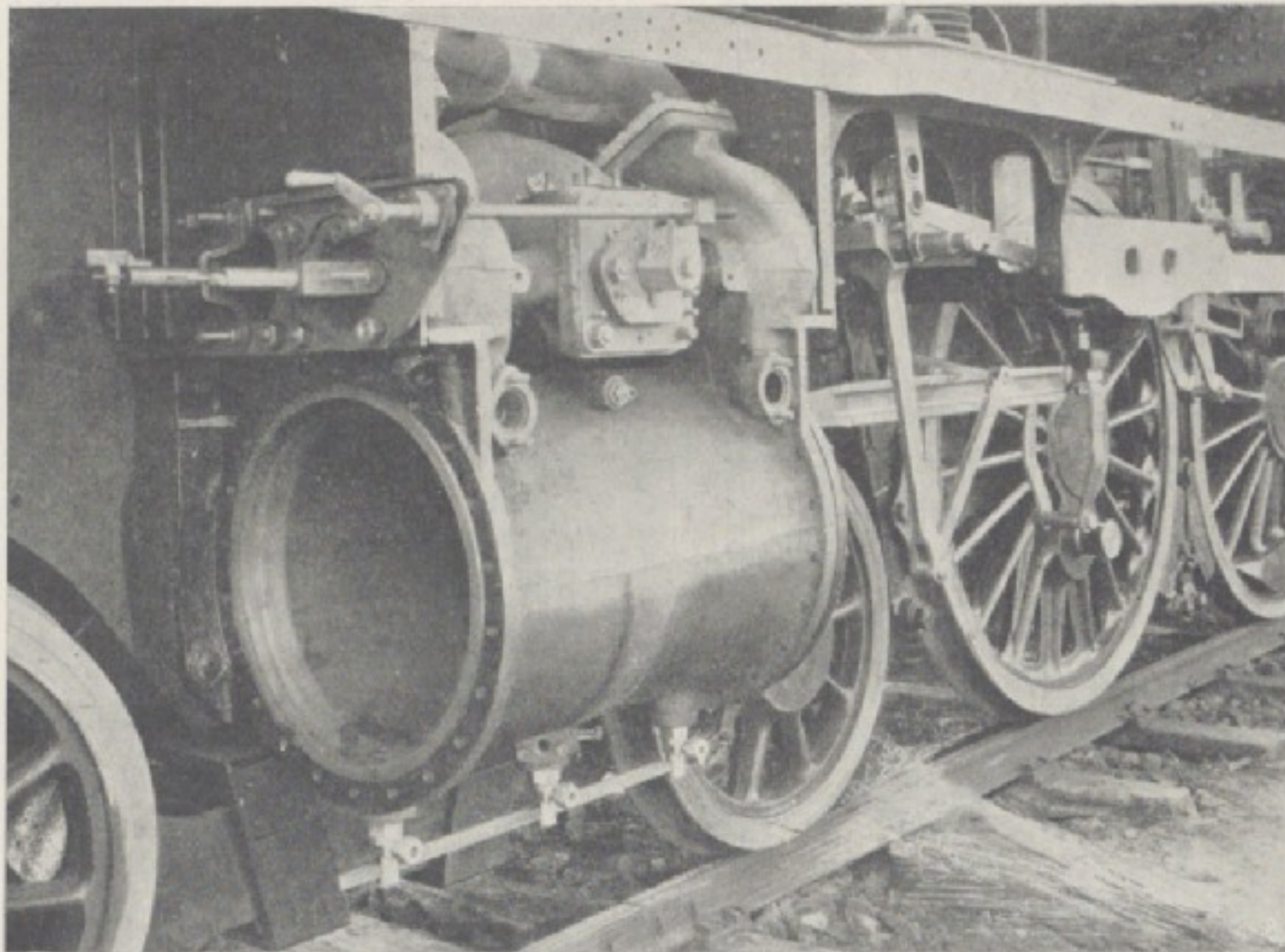
Fig. 7. Ustawianie zaworowego stawidła wewnętrznego na par. Ok22.
