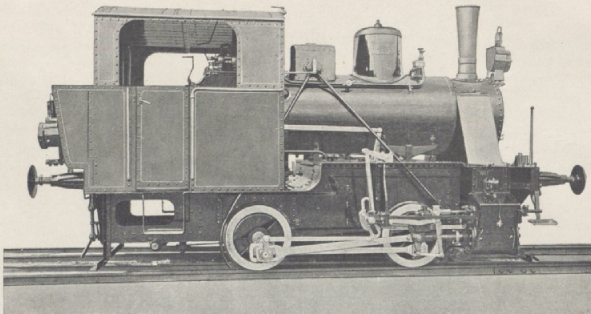
Fig. 15. Tendrzak 0—2—0 moc 100 KM normalnotor.
