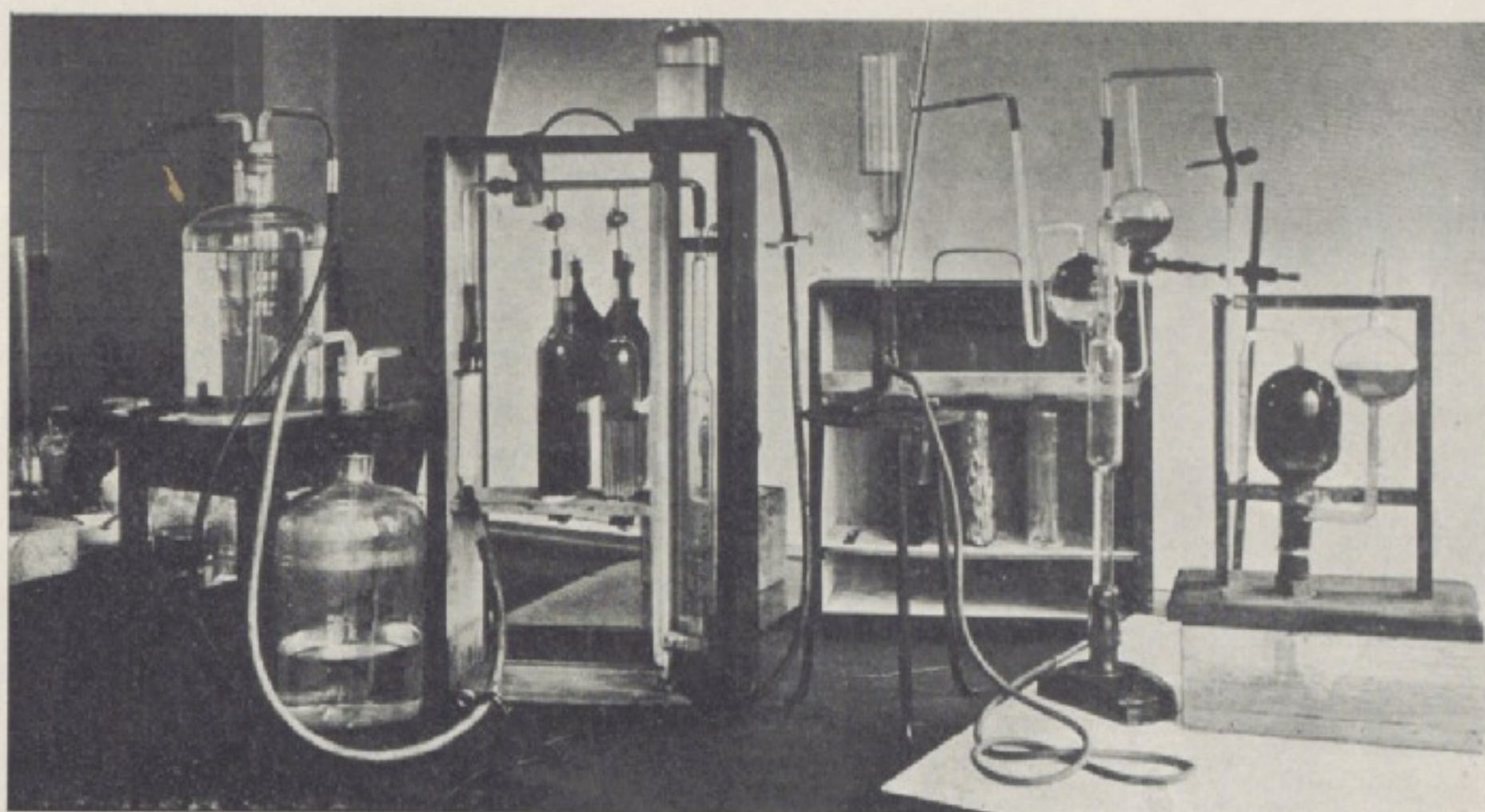
Fig. 1. Przyrządy, używane do badania tlenu.
