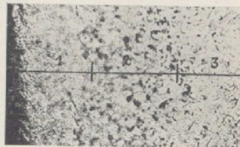
Mikrofotogr. 2. \times 50 (25).
