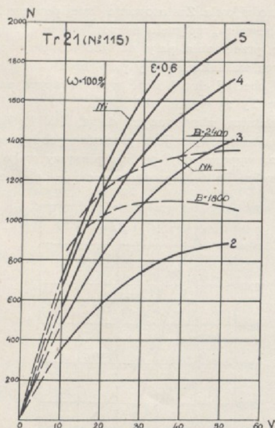
Fig. 10. Krzywe mocy parowozu Tr 21.
