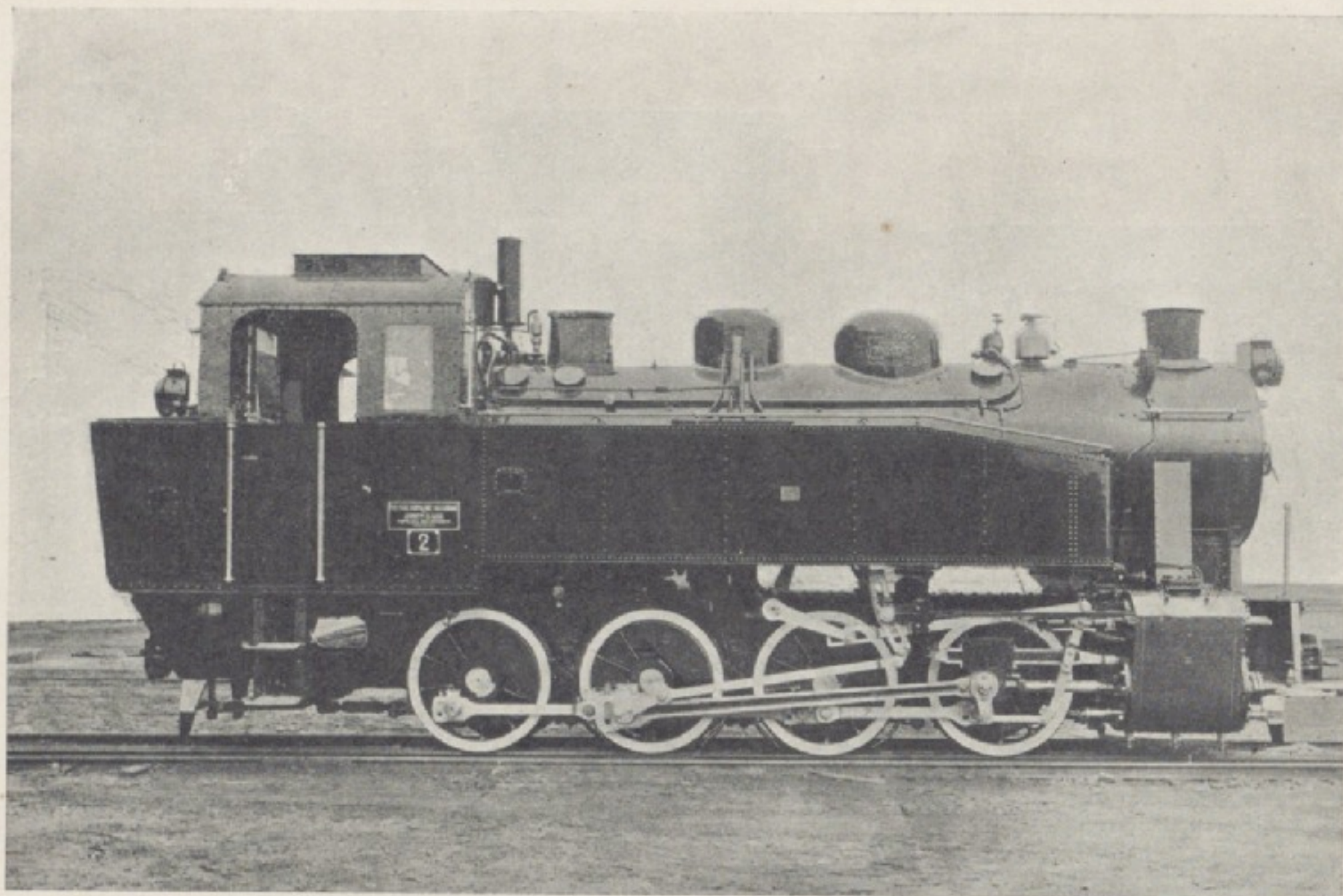
Fig. 11. Tendrzak 0—4—0 moc 400 KM szer. toru 1000 m/m na parę przegrzaną.
